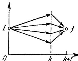
Рис. 23. К прямому уравнению.
