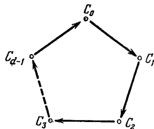
Рис. 38. Движение по циклическим подклассам.
