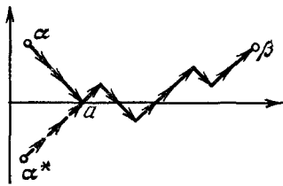
Рис. 17. К принципу отражения.
