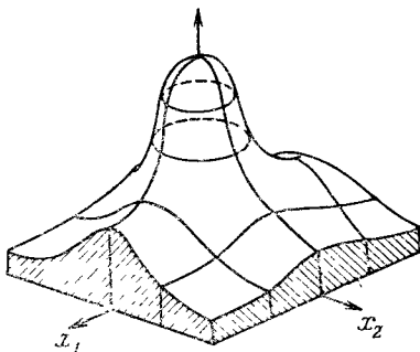
Рис. 28. Плотность двумерного нормального распределения.
